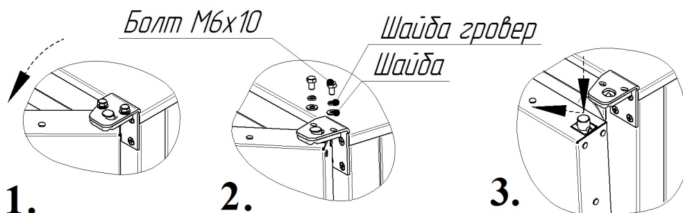
Рис. 10 Снятие двери.
