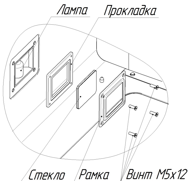
Рис. 9. Замена лампы освещения и прокладки
