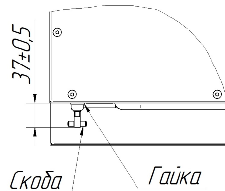
Рис. 8. Регулировка замкового устройства в КЭП-10П
