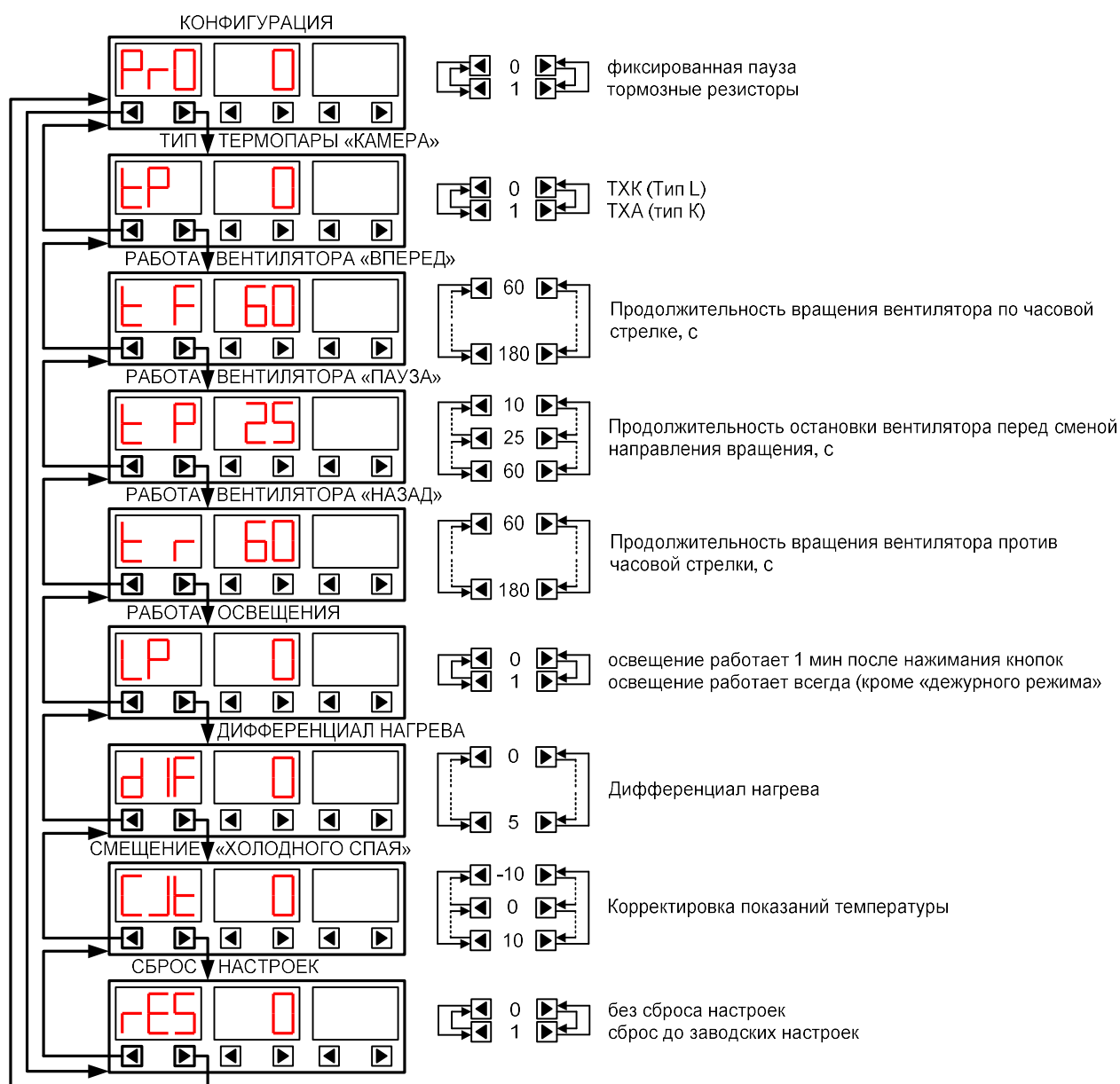
Рис.11 Настройка контроллера
