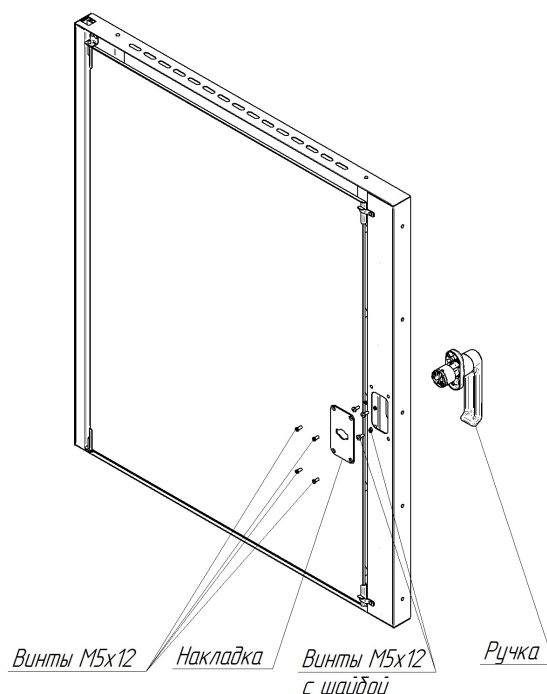
Рис. 6. Замена ручки в КЭП-10П
