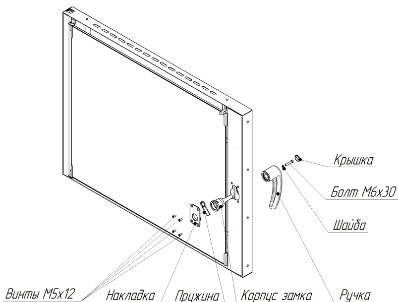
Рис. 5. Ремонт замкового устройства в КЭП-6П
