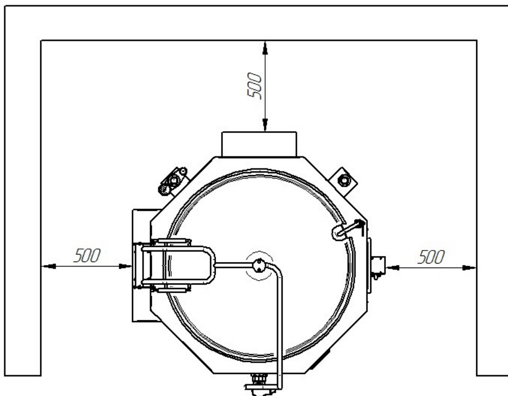
Рисунок 2 Установка котла
