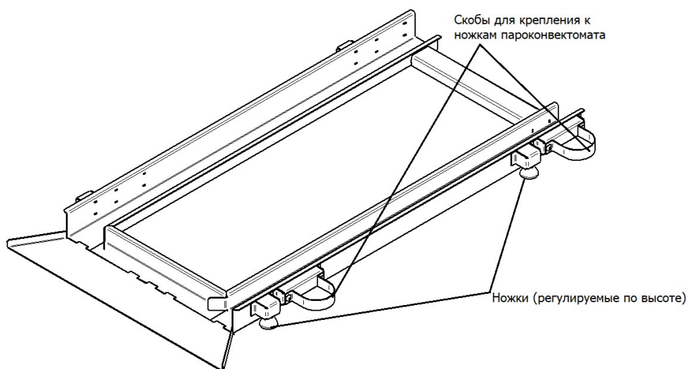
Подставка ПТП-20
