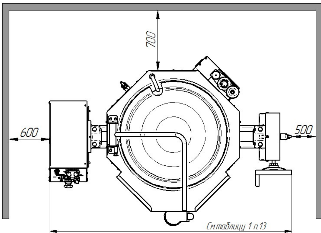
Рис. 4. Установка котла
