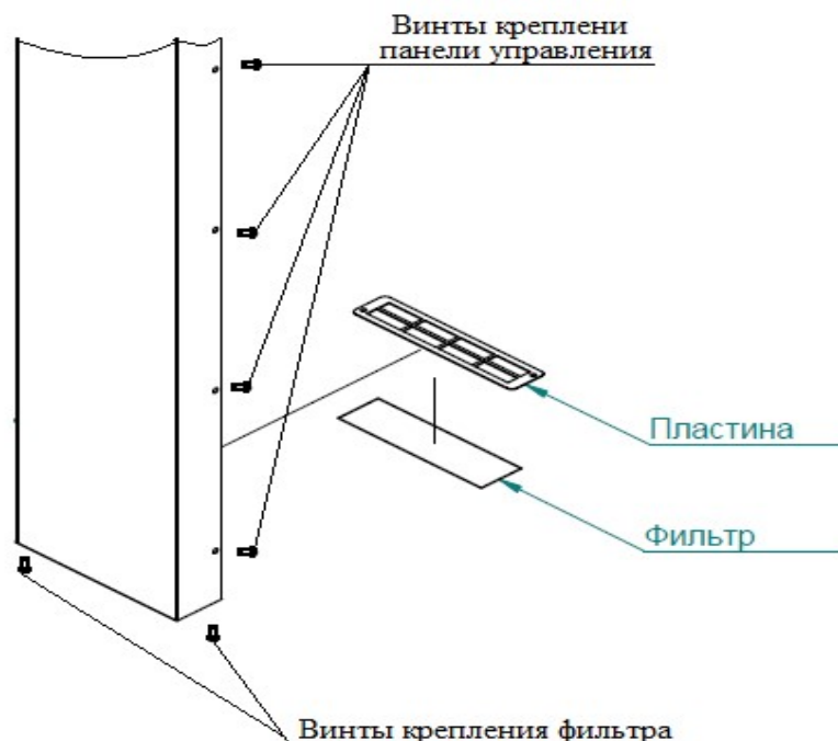
Рис.20. Замена фильтра
