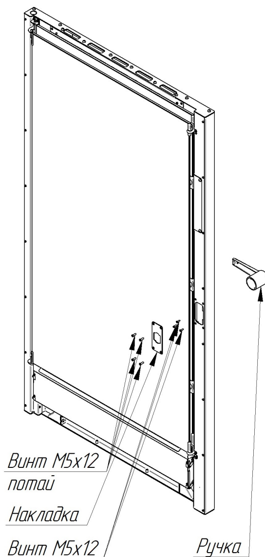
Рис. 17. Ремонт замкового устройства
