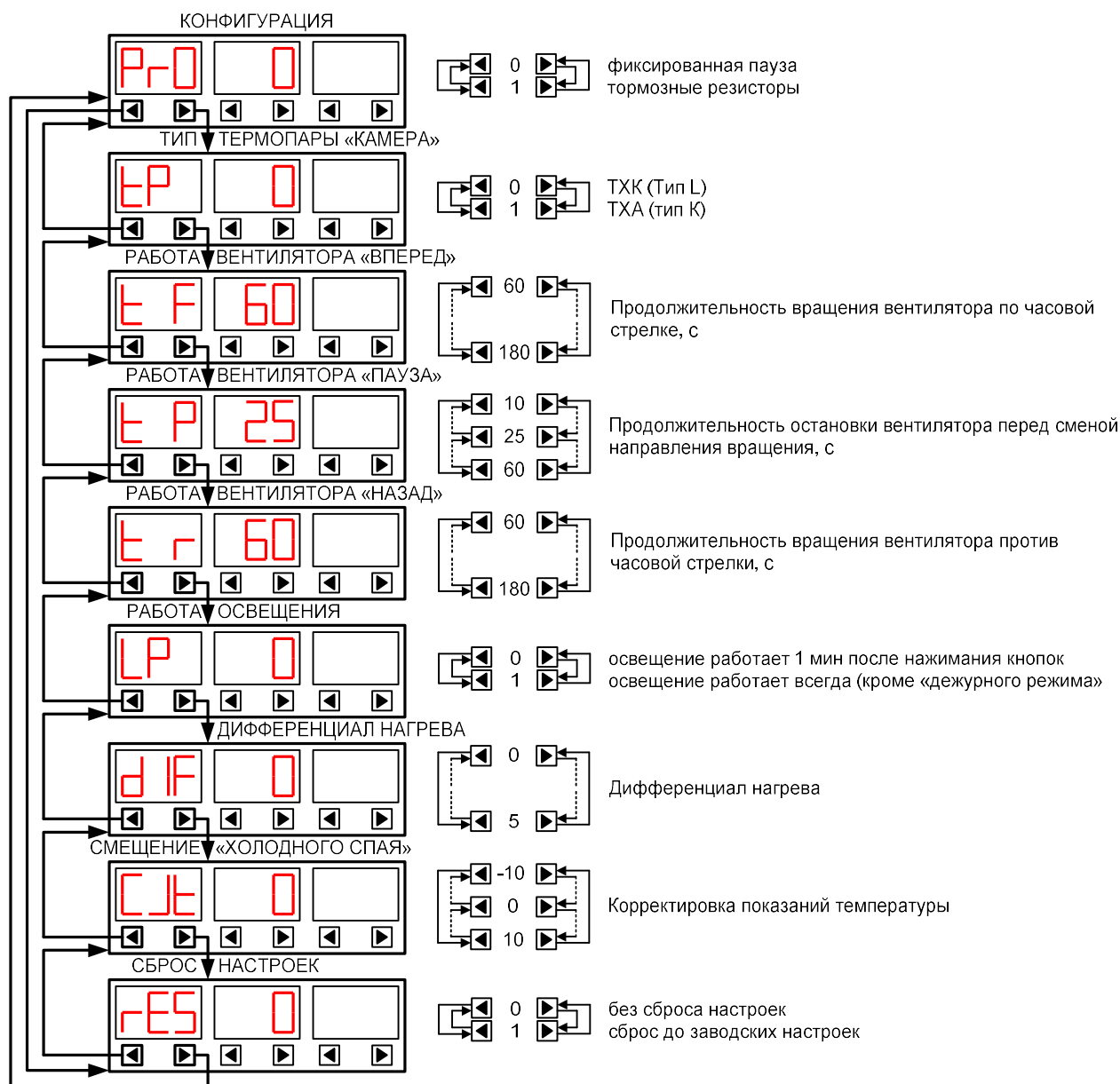
Рис.5 Настройка контроллера
