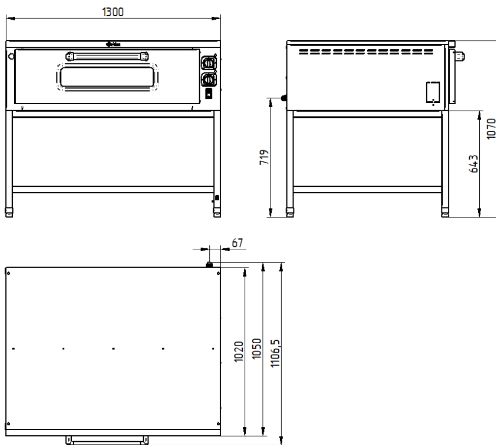
Рис. 1. Общий вид ЭШП-1-01.
