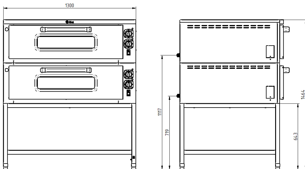
Рис. 2. Общий вид ЭСП-2-01.
