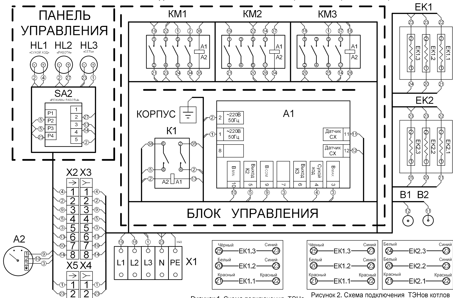
Рисунок 1. Схема подключения ТЭНа котлов КПЭМ-60/7Т, КПЭМ-60/9Т
