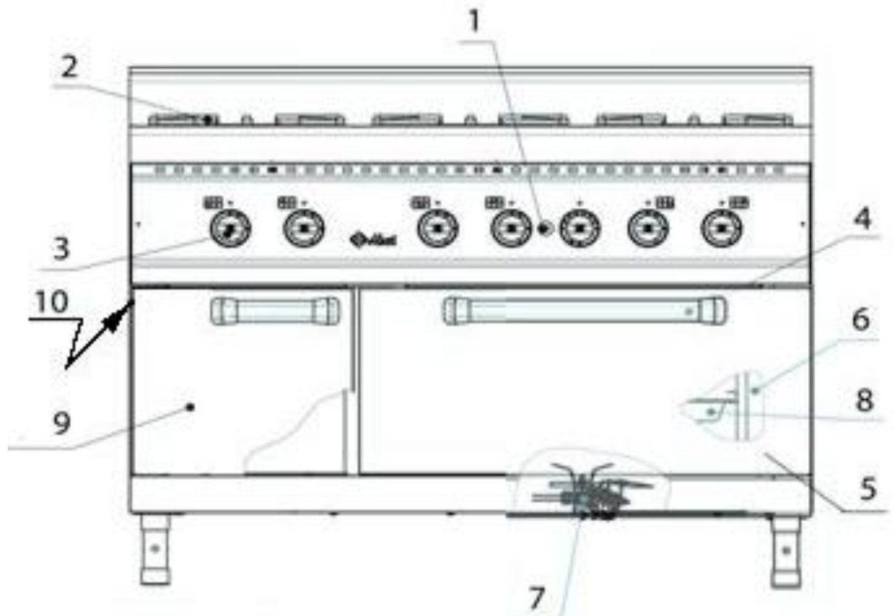
Рис. 1. Плита ПГК-69ЖШ-II-A
