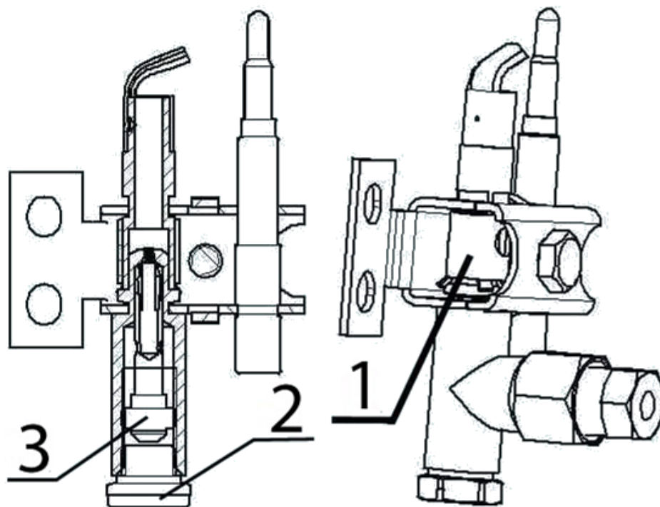
Рис. 11 Запальная горелка стола (пилот)
