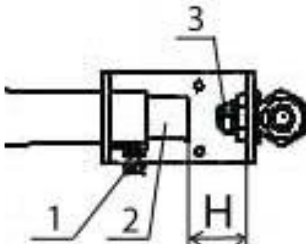
Рис. 10 Горелка духовки
