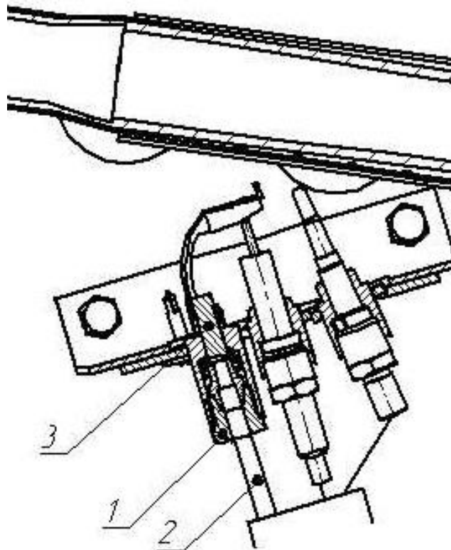
Рис.12 Запальная горелка духовки (пилот)
