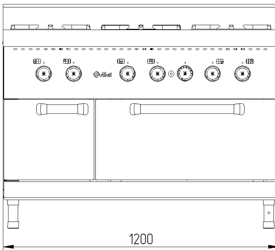
Габаритные размеры газовой плиты ПГК-49ЖШ-П-А
