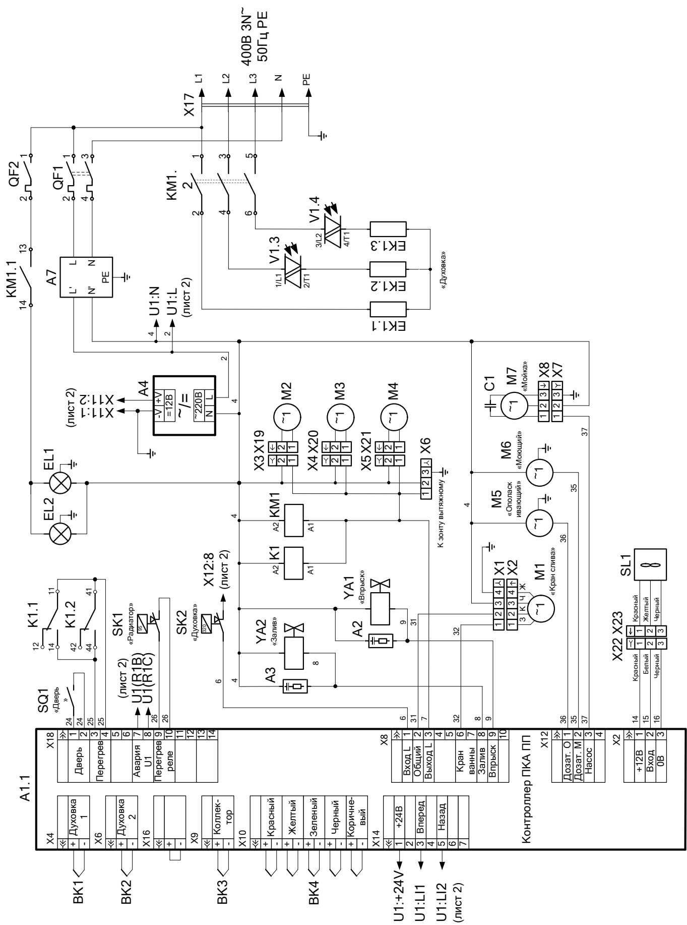
СХЕМА ЭЛЕКТРИЧЕСКАЯ ПРИНЦИПИАЛЬНАЯ ПКА6-1/1ВП2, ПКА10-1/1ВП2
