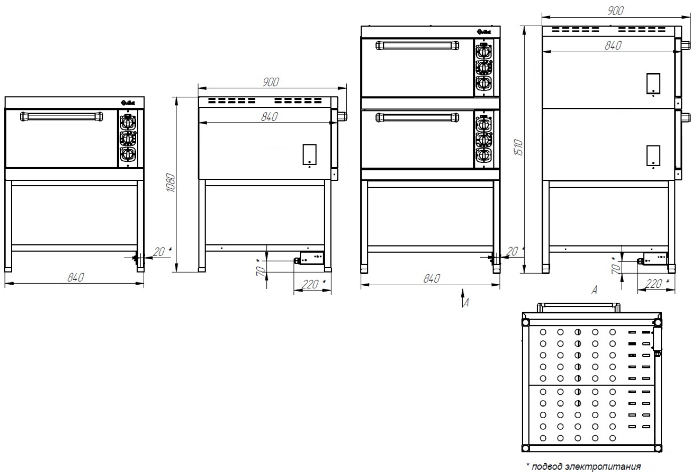
Рис. 6 Шкаф жарочный ШЖЭ-1-Э, ШЖЭ-2-Э
