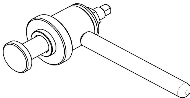
Рис. 11. Приспособление для запрессовки манжет(11000001333).
