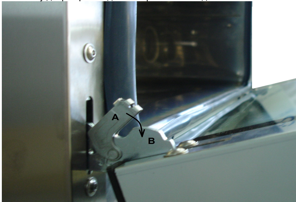
Рис. 3 Снятие двери.
