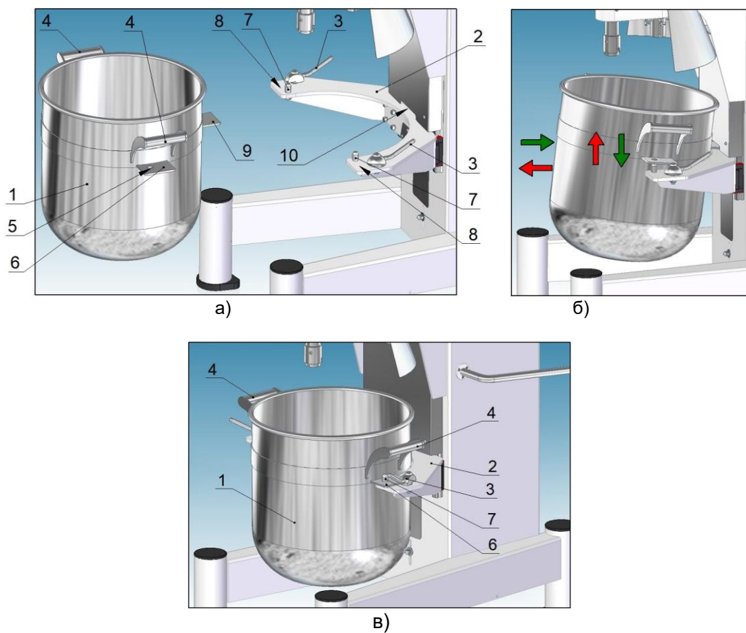
Рис. 5 Установка/извлечение дежи
