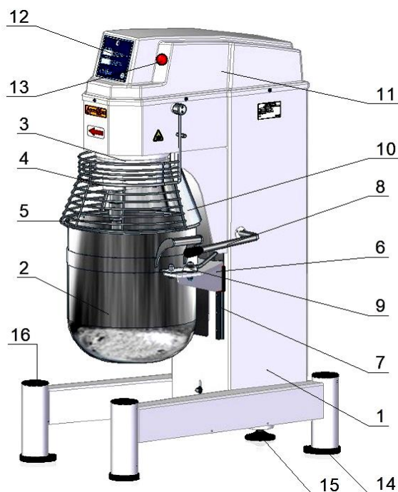
Рис. 1 Устройство миксера
