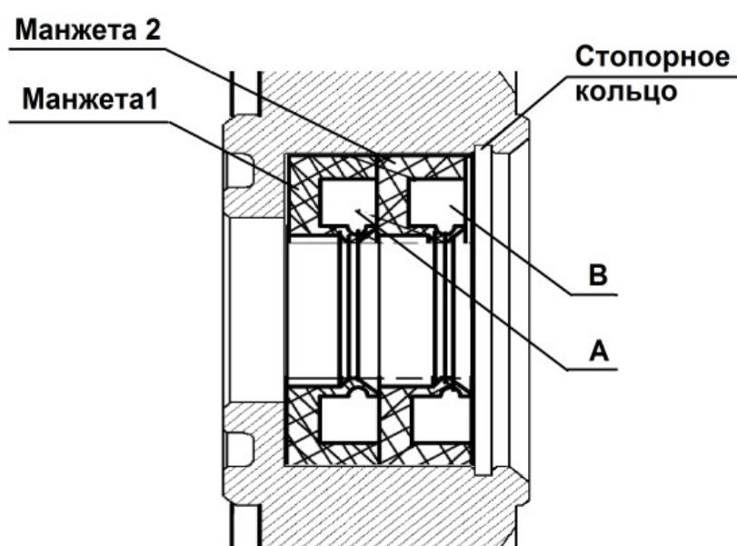
Рис. 10. Схема установки манжет.
